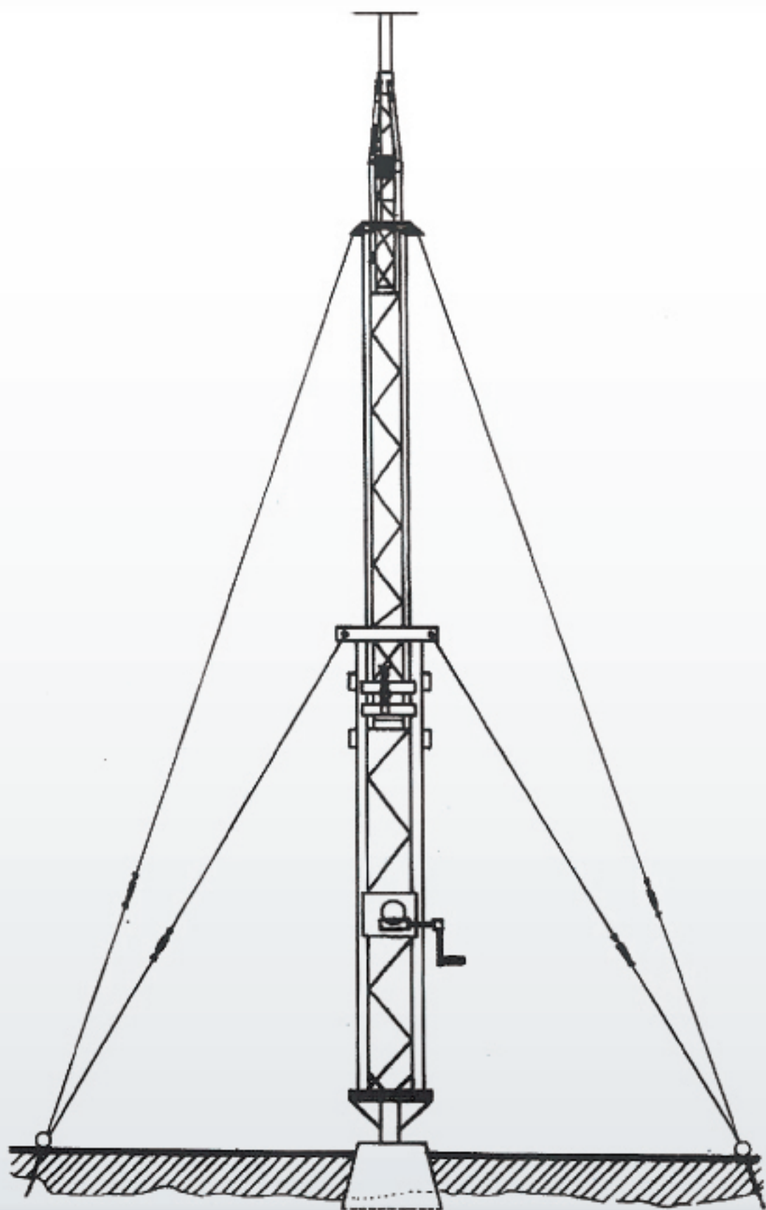
TRALICCIO TELESOPICO
