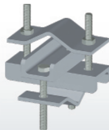
ZANCA PER RADIATORI
