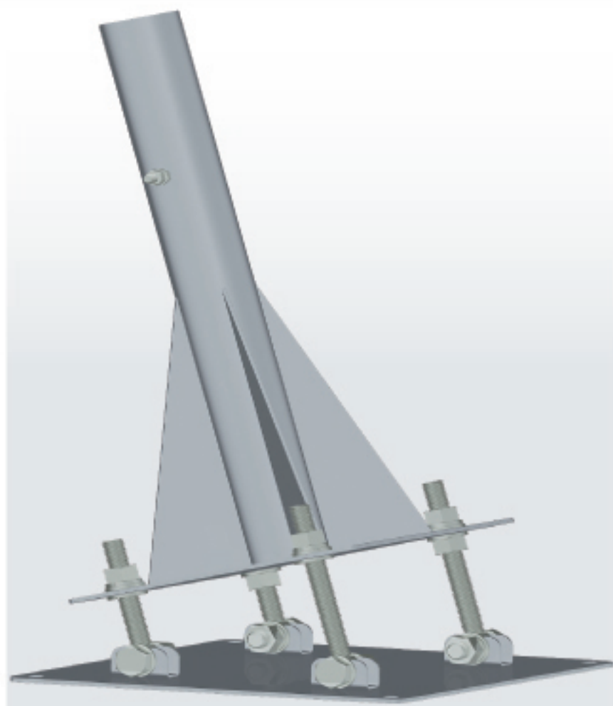
SISTEMA PER L'INSTALLAZIONE PERPENDICOLARE DI SOSTEGNI PER PARABOLA E ALTRI USI
